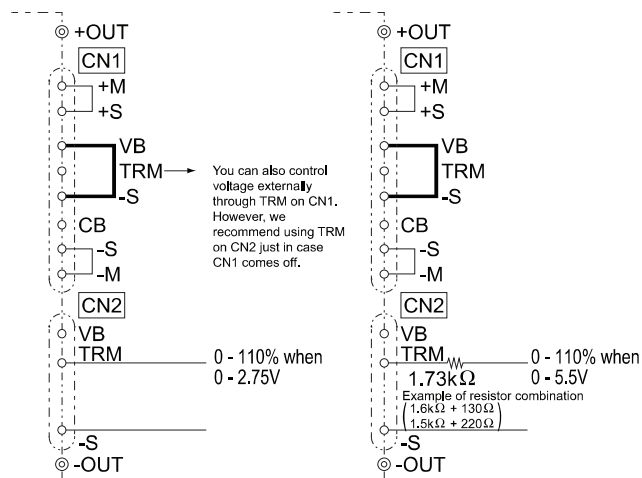
Fig.2.1 Wiring 1
